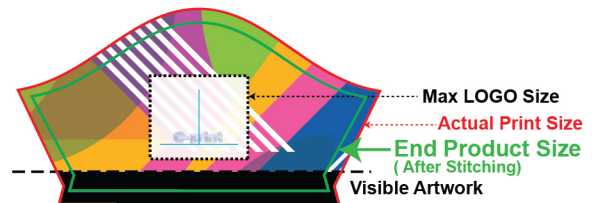
S.SLEEVE LEFT
